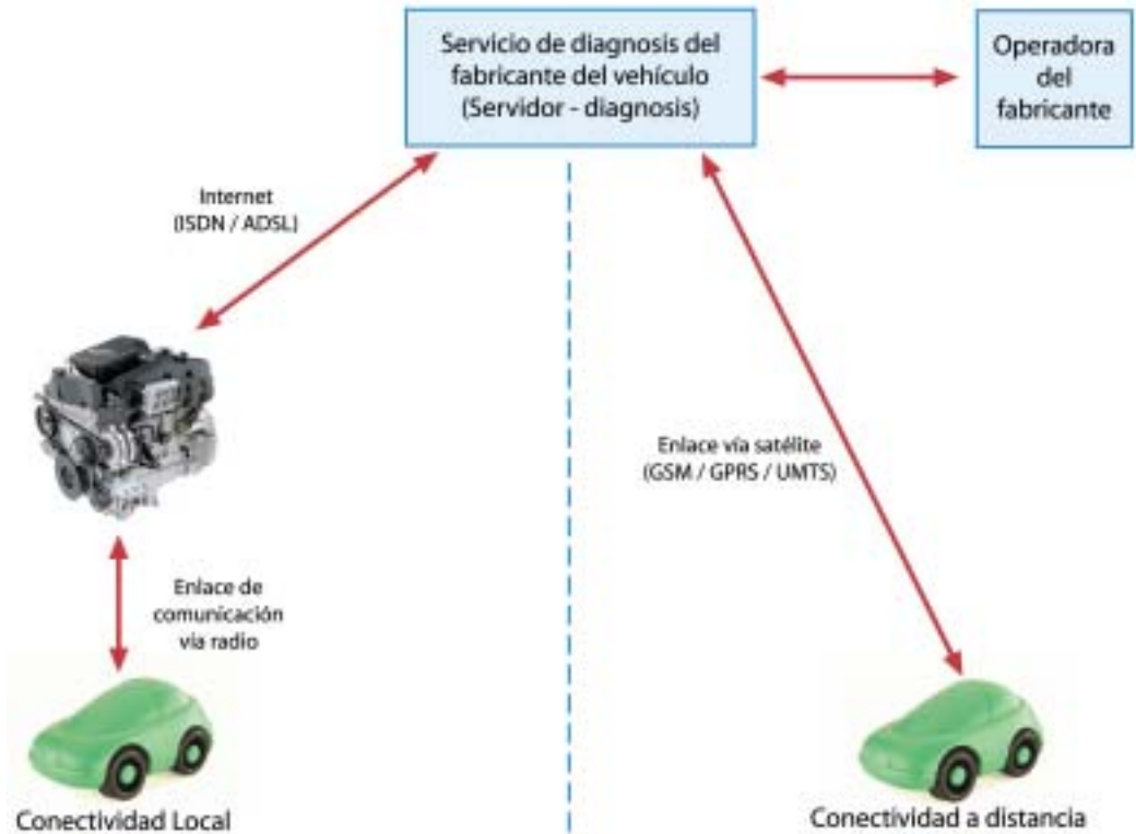
Figura 2.4 Diagrama de bloques ilustrativo de la diagnóstico remoto (off- line)
