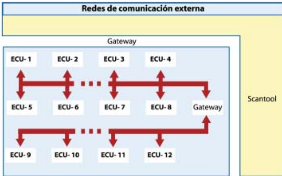
Figura 2.16 Ejemplo de sistemas de comunicación entre los ECU's y del vehículo con el mundo exterior.
