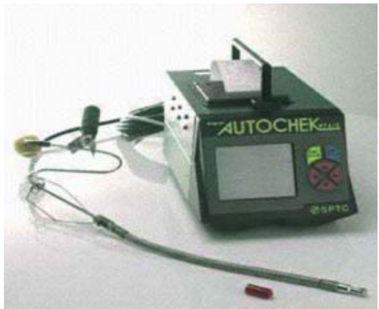
Figura 2.2 Ejemplo de equipo con sensores externos utilizados en la diagnos is externa aplicada a la detecci3n de fallos en los autom3viles
