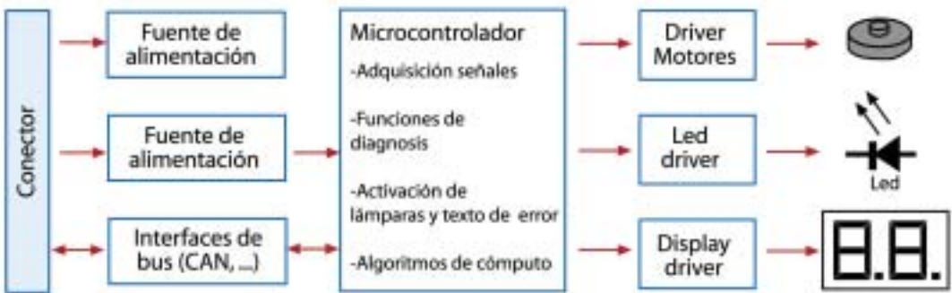
Figura 3.21 Esquema de un panel de instrumentación (instrument cluster) típico de automóvil.
