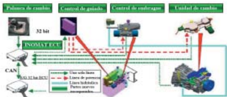
Figura 4.21 Diagrama de bloques general del sistema INOMAT-II
