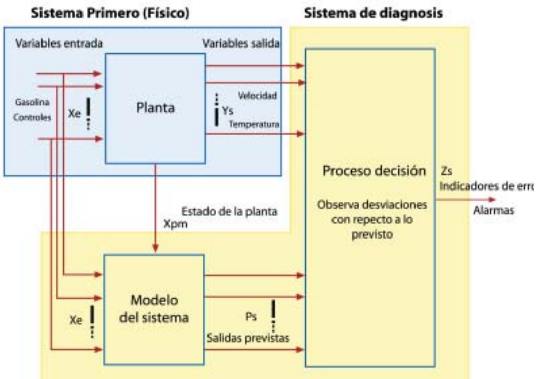
Figura 3.24 Esquema genérico de la estrategia de diagnosís interna del automóvil.
