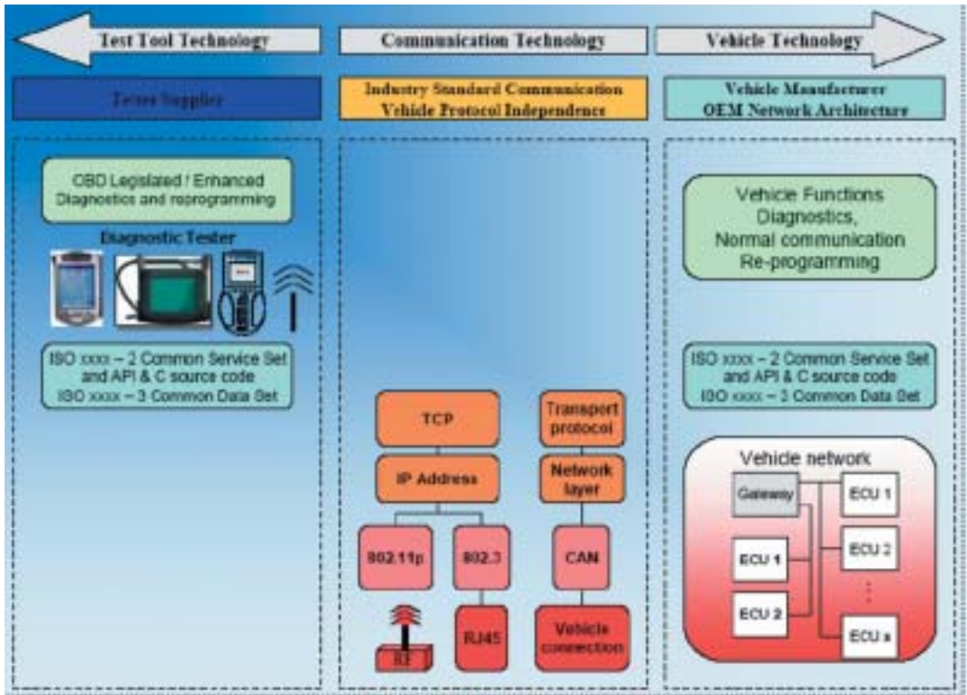
Figura 4.68 Distintos protocolos de comunicación de los dispositivos involucrados en la diagnosis
