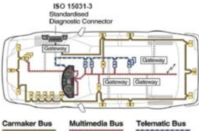
Figura 3.15 Ejemplo de interconexión entre redes de comunicación de un vehículo.
