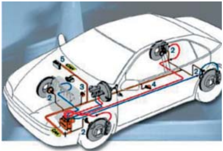
Figura 4.13 Elementos asociados al ESP
