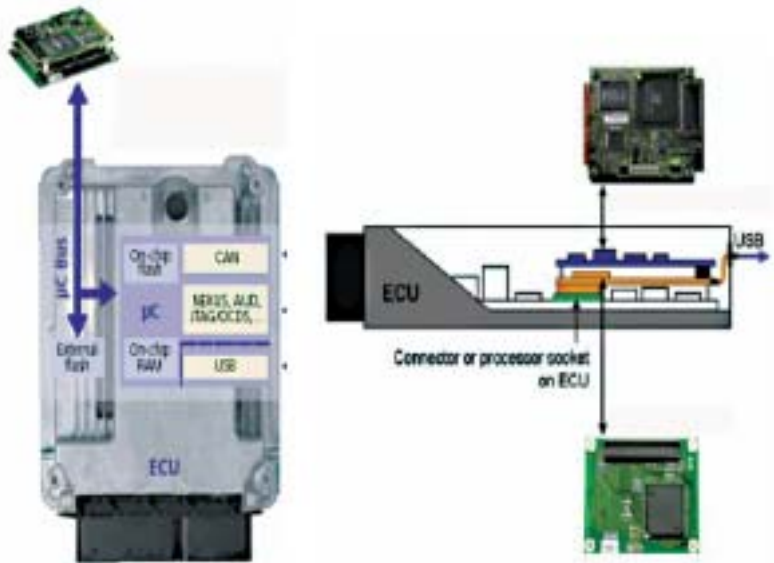
Figura 4.36 Ejemplo de ECU real, con las diferentes etapas electrónicas que incluye.
