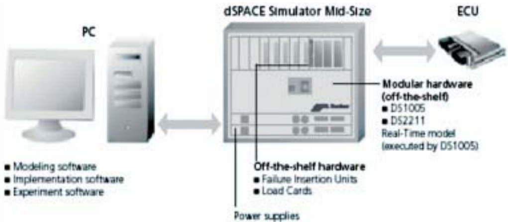
Figura 4.31 Ejemplo de prueba de un ECU en un sistema de emulación (Hardware in the Loop)
