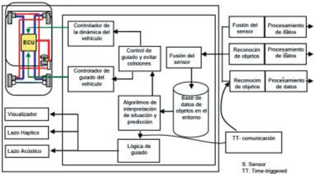
Figura 4.63 Elementos integrados en el emulador para diagnóstico y calibración de un ECU en condiciones de evitación de colisiones.
