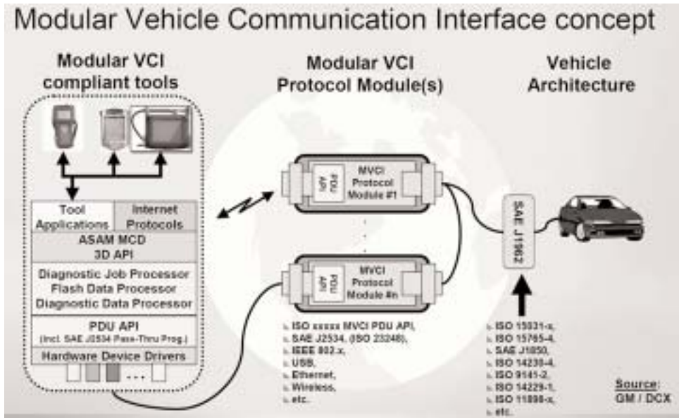
Figura 4.67 Interconexión modular entre equipos de diagnóstico y el sistema electrónico del vehículo.
