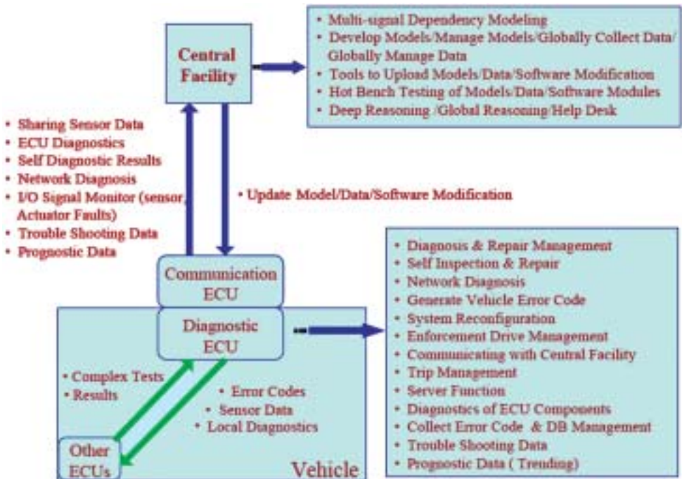
Figura 4.56 Funciones e intercambio de información entre agentes de la arquitectura de diagnóstico distribuida.
