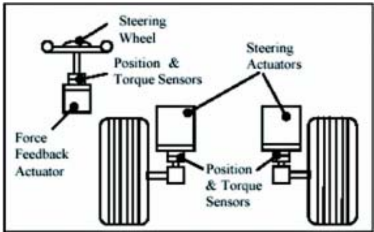
Figura 4.24 Sensores y actuadores utilizados en el sistema de dirección por cable (steer-by-wire).
