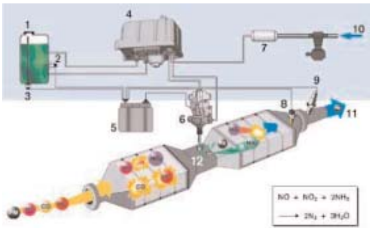
Figura 4.18 Catalizador SCR
