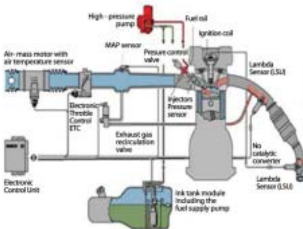
Figura 3.8 Ejemplo de ECU: contexto de aplicación y tarjeta electrónica de la unidad de control.
