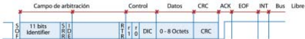
Figura 3.18 Formato de mensajes utilizado en bus CAN.
